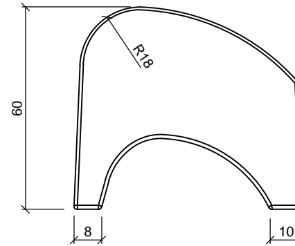
PERFIL / RIGHT SIDE
