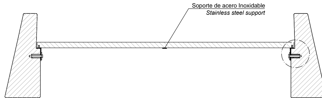
SECCIÓN A-A' / SECTION A-A'
